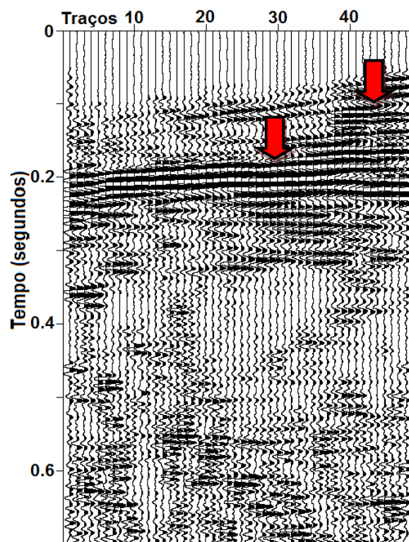
Figura 11 - Conjunto de receptor comum, Colônia, componente H radial. Aplicados filtro PB, Filtro de polarização, filtro FK e Ganho AGC. Os eventos que apresentam velocidades da onda PP estão indicados com seta vermelha.
