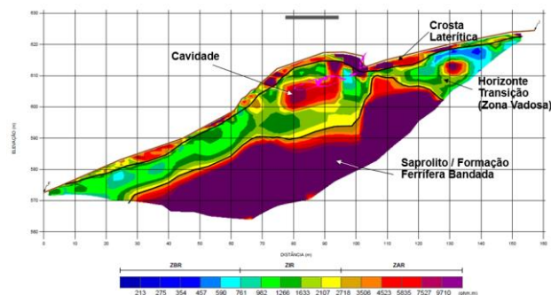
Figura 10 - Seção Eletroresistividade sobre a cavidade N4E-0026. Notar a diferenciação dos padrões resistivos em 3 horizontes, que corroboram com os perfis lateríticos ferruginosos da região.
