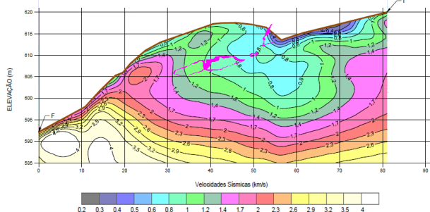
Figura 5 - Seção Sísmica de Refração (SR) com até 42 m de profundidade sobre a cavidade N4E-0026. A zona ondulada com baixas velocidades está associada a presença da cavidade.
