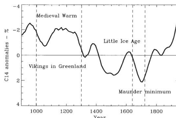
Figura 01 – Associação entre a atividade solar (representada pelas anomalias de 14 C) e os longos períodos de variação climática extrema, Medieval Warm (1000 – 1300) e Maunder Minimum (1645 – 1715). Adaptada de Svensmark (2000).
