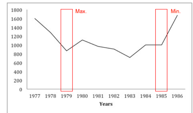
Figura 04 – Índice pluviométrico médio anual na cidade de Martins durante o ciclo solar 21.
