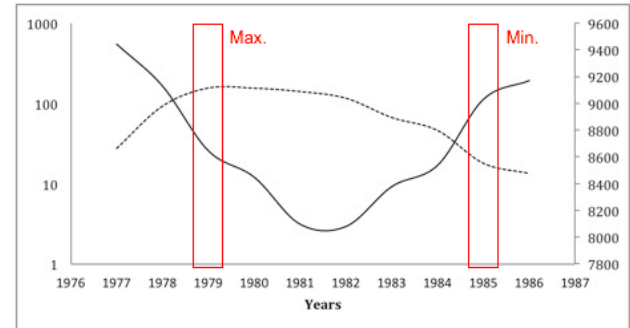
Figura 03 – Valores anuais de manchas solares (curva tracejada) e raios cósmicos (curva contínua) durante o ciclo solar 21.
