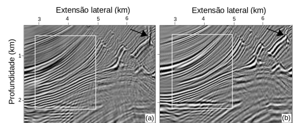
Figura 9: Efeito do janelamento das PSFs sobre a imagem migrada deconvolvida. (a) Sem janelamento Nuttall radial. (b) Com janelamento Nuttall radial.
