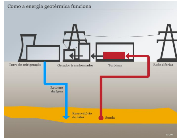
Figura 9: Desenho esquemático de uma central geotérmica
