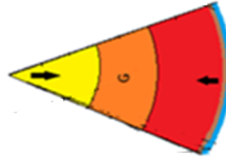
Figura 5: A Terra há 600 MA, após perder um volume de massa varias vezes a atual. A massa perdida espalhou-se como asteróides e cometas pelo Sistema Solar e os que não conseguiram velocidade orbital caíram no Sol.
