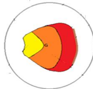
Figura 6: Grande parte da água ficou em estado de vapor e cobriu completamente o planeta.
