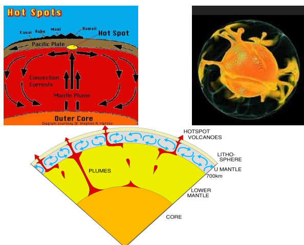
Figura 1: Três Exemplos de interpretação de Mantle Plumes e Hotspots
