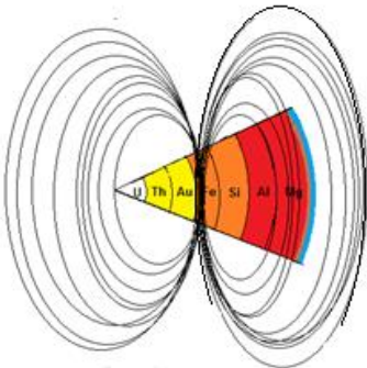
Figura 4: O campo magnético foi instantaneamente formado pela calota de Ferro, o ímã inicial.
