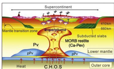
Figura 1: Três Exemplos de interpretação de Mantle Plumes e Hotspots
