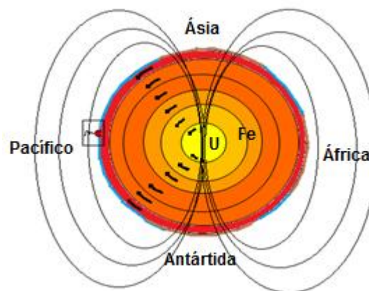
Figura 11: O movimento quase horizontal e contínuo de parte da camada ou esfera de Ferro gera o atrito que mantém o campo magnético da Terra. Não há diferença de velocidade angular entre as esferas do manto.
