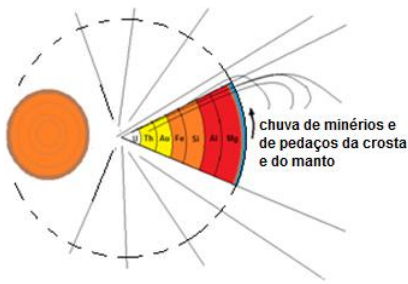
Figura 3: A massa que sobrou da Terra tinha aspecto quase cônico.
