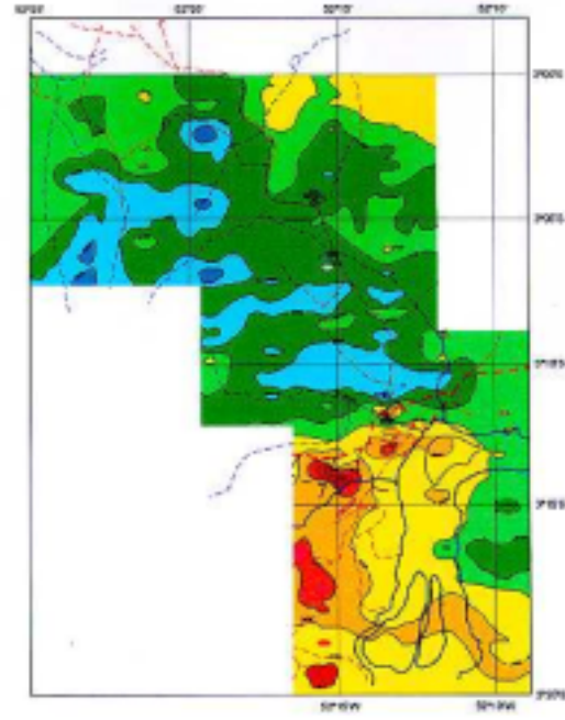
Figura 3 Mapa de isogamas do campo magnético total
