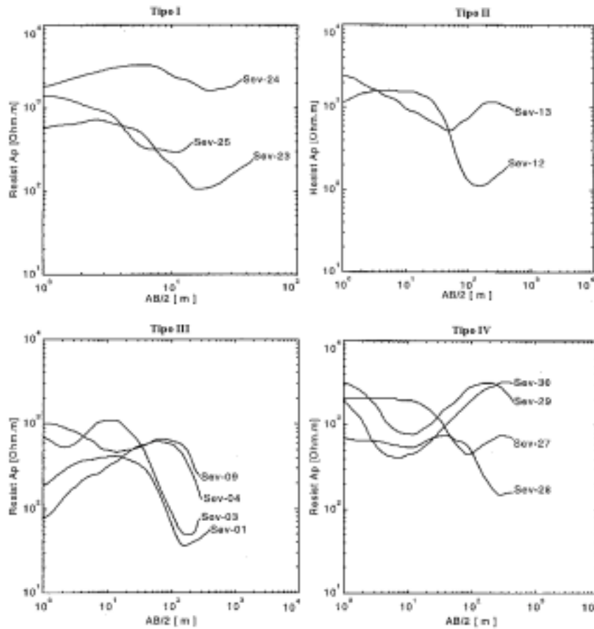
Figura 4 Família de curvas de sondagem obtidas
