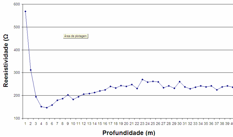
Gráfico 3: Valores de resistividade aparente dos CEHs efetuados às profundidades de 10,0m , 20,0m e 30,0m, no Local P3, linha L0
