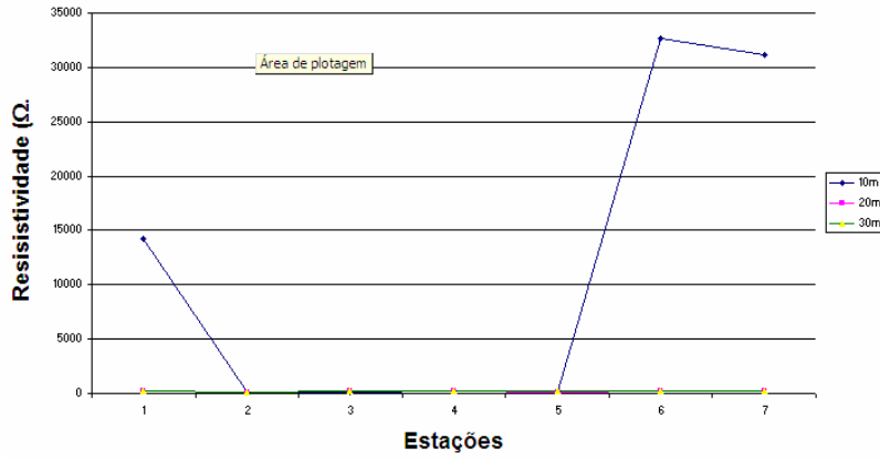
Gráfico 1: Valores de resistividade aparente dos CEHs efetuados às profundidades de 10,0m , 20,0m e 30,0m, no Local P2
