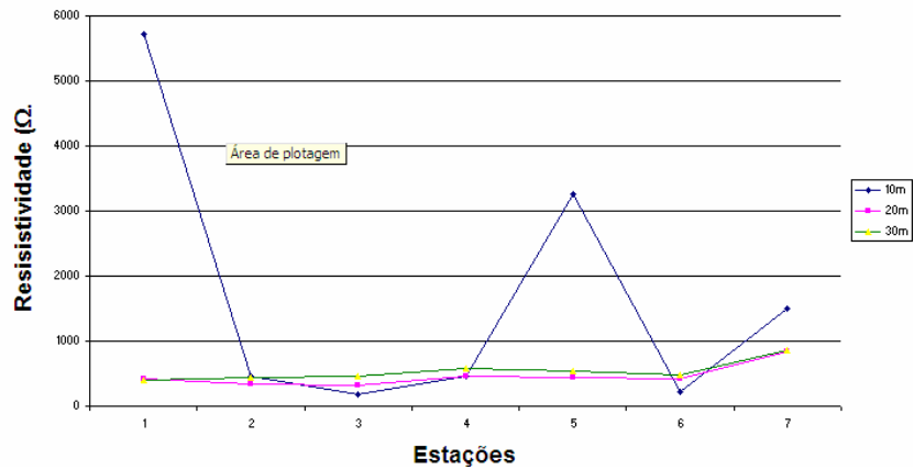
Gráfico 5: Valores de resistividade aparente dos CEHs efetuados às profundidades de 10,0m , 20,0m e 30,0m, no Local P3, linha L2
