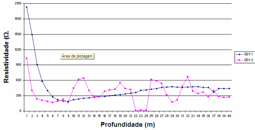
Gráfico 7: Valores de resistividade aparente referentes às SEV 1 e SEV 2, no Local P3
