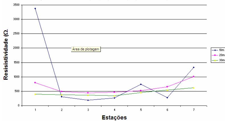
Gráfico 6: Valores de resistividade aparente dos CEHs efetuados às profundidades de 10,0m , 20,0m e 30,0m, no Local P3, linha L3
