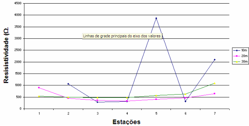
Gráfico 4: Valores de resistividade aparente dos CEHs efetuados às profundidades de 10,0m , 20,0m e 30,0m, no Local P3, linha L1
