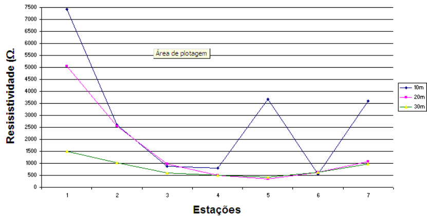
Gráfico 3: Valores de resistividade aparente dos CEHs efetuados às profundidades de 10,0m , 20,0m e 30,0m, no Local P3, linha L0
