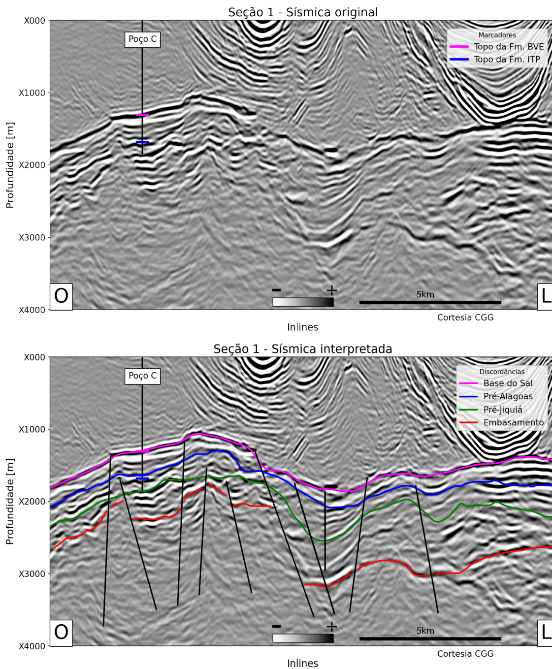
Figura 46 – Seção sísmica 1 que passa pelo Poço C, com os marcadores do poço (acima) e a interpretação das discordâncias e das principais falhas no intervalo do pré-sal (abaixo).
