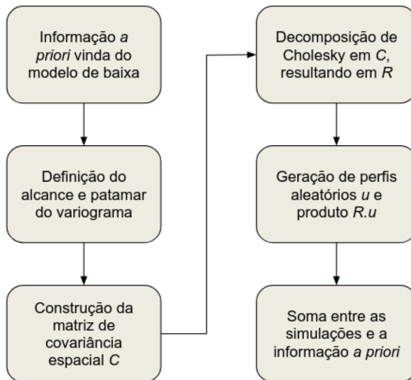
Figura 26 – Fluxo adotado para a construção das simulações estocásticas espacialmente correlacionadas verticalmente.
