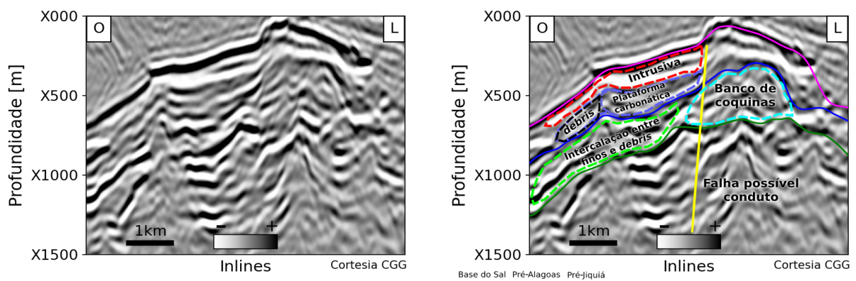
Figura 47 – Intervalo leste da Seção sísmica 1 que mostra a intrusão ígnea no dado original (esquerda) e no dado interpretado (direita). A escolha das cores da interpretação foi arbitrária.
