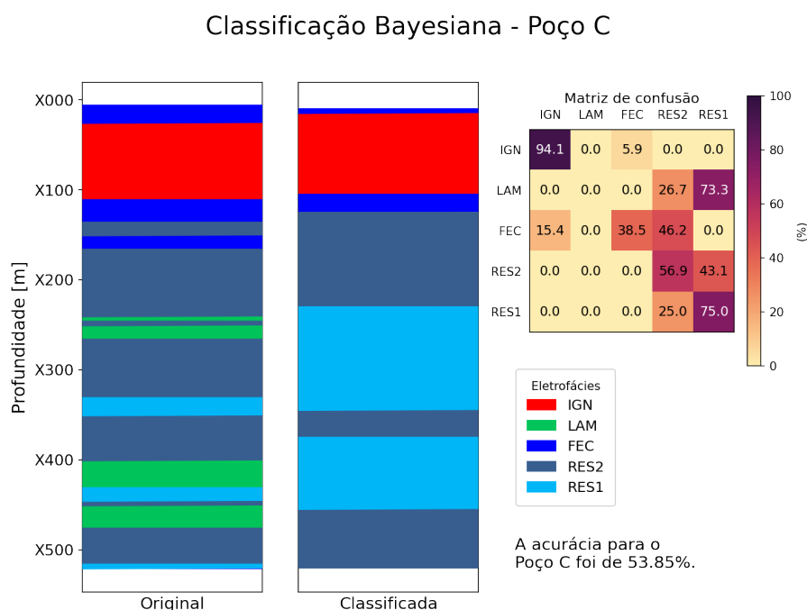
Figura 64 – Eletrofácies originais do Poço C e a extraída do volume classificado na posição do poço. Além disso, é mostrada a matriz de confusão e a acurácia estimada neste intervalo.
