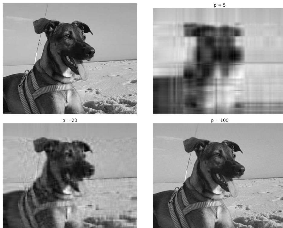
Figura 11 – Decomposição SVD na imagem de um cachorro. No canto superior esquerdo é mostrada a imagem original. No canto superior direito é mostrada a imagem quando p = 5 . No canto inferior esquerdo é para quando p = 20 e no canto inferior direito é no caso em que p = 100 . Nota-se uma melhora na reprodução da imagem original com um maior número de valores singulares retidos.
