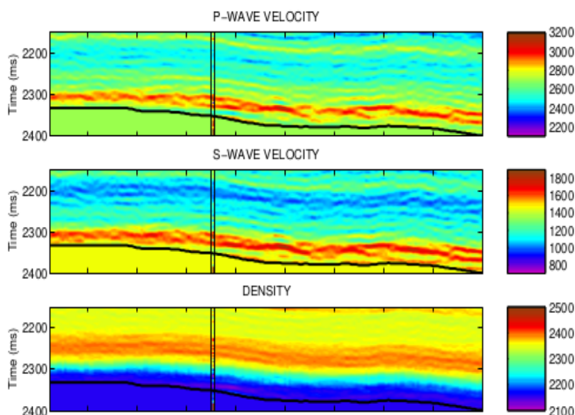
Figura 18 – Solução máxima a posteriori de uma inline do Campo de Sleipner Øst, no Bloco 15/9 da Noruega, mostrando o resultado da inversão Bayesiana linearizada para um dado pré-empilhamento com a velocidade compressional (acima), a velocidade cisalhante (meio) e a densidade (abaixo). Fonte: Buland e Omre (2003).
