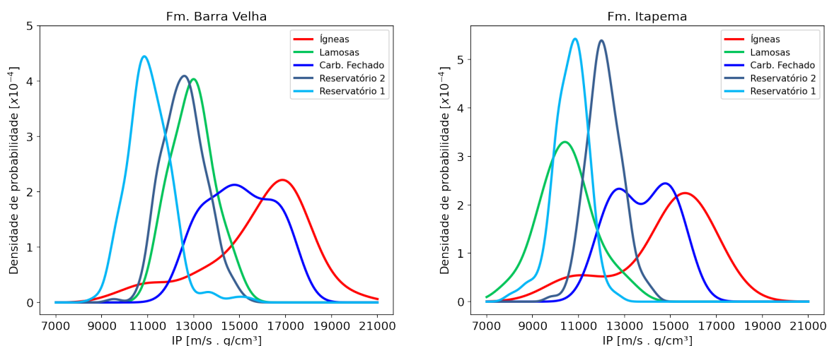
Figura 38 – Funções de densidade de probabilidade da verossimilhança condicional estimadas usando a estimativa de densidade do kernel para as eletrofácies reservatórios 1, reservatórios 2, carbonatos fechados, lamosas e ígneas nas formações Barra Velha (esquerda) e Itapema (direita).
