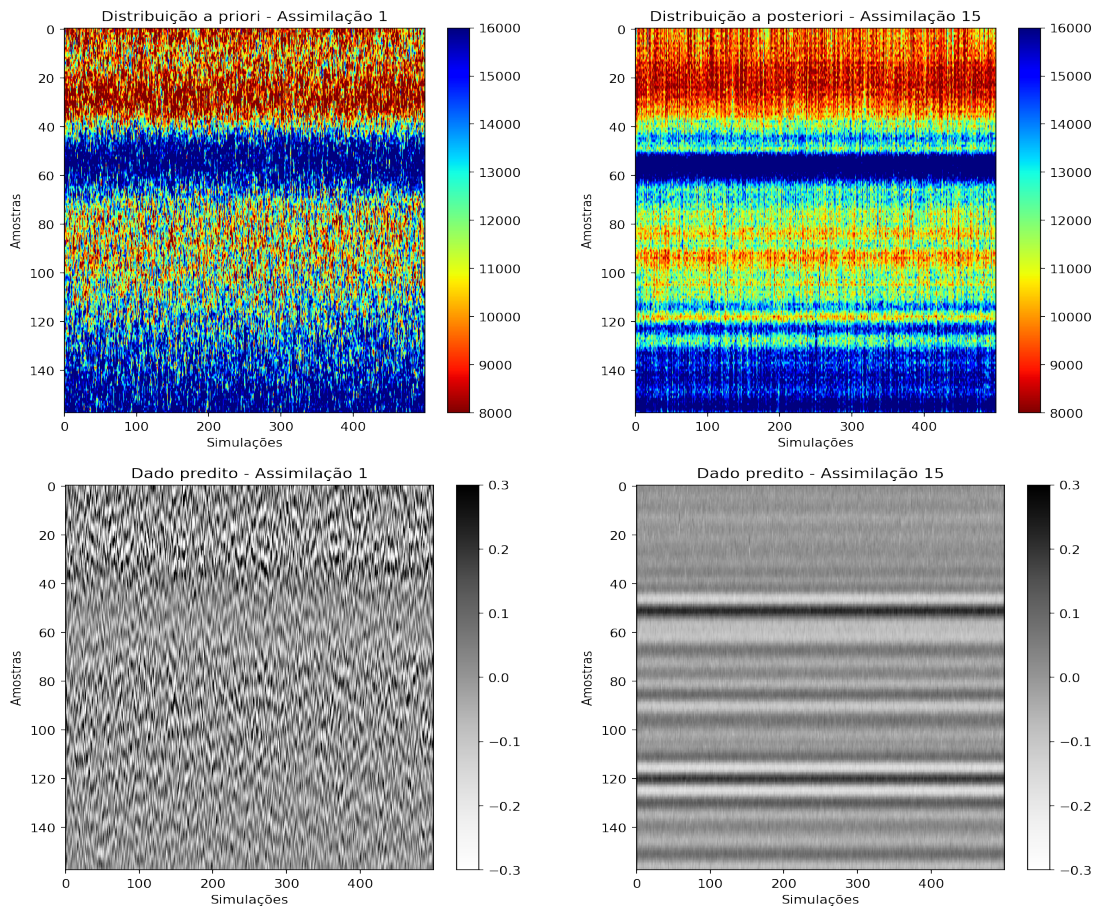
Figura 35 – Conjuntos de impedância acústica (acima) e sua modelagem direta em amplitude (abaixo) antes da primeira iteração (esquerda) e após a última iteração (direita).
