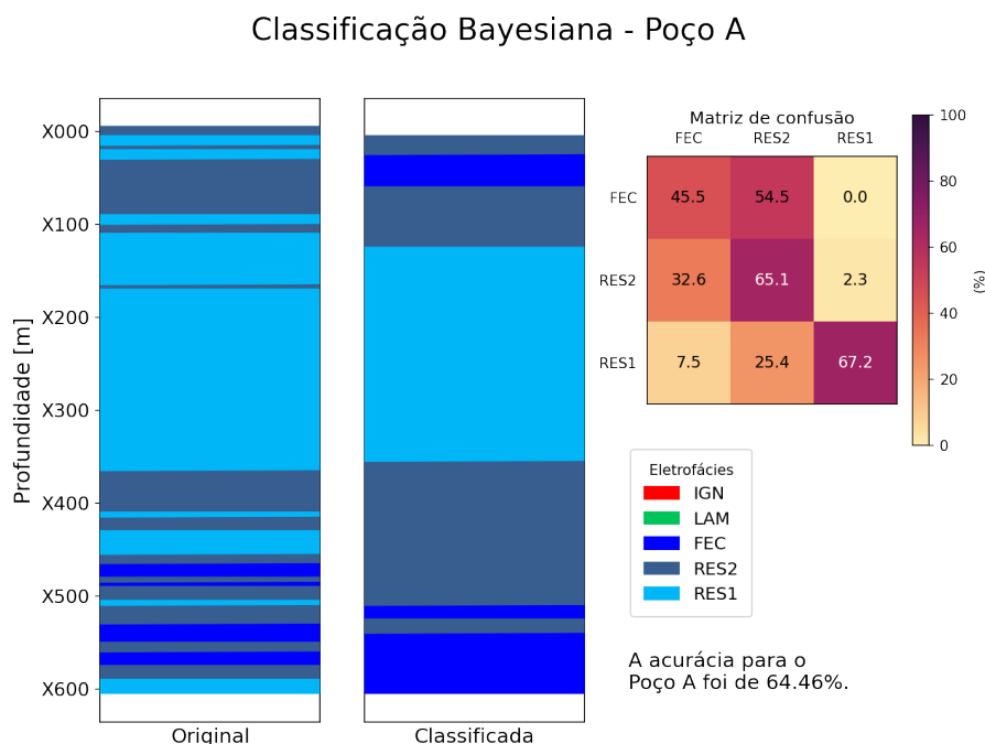
Figura 66 – Eletrofácies originais do Poço A e a extraída do volume classificado na posição do poço. Além disso, é mostrada a matriz de confusão e a acurácia estimada neste intervalo.
