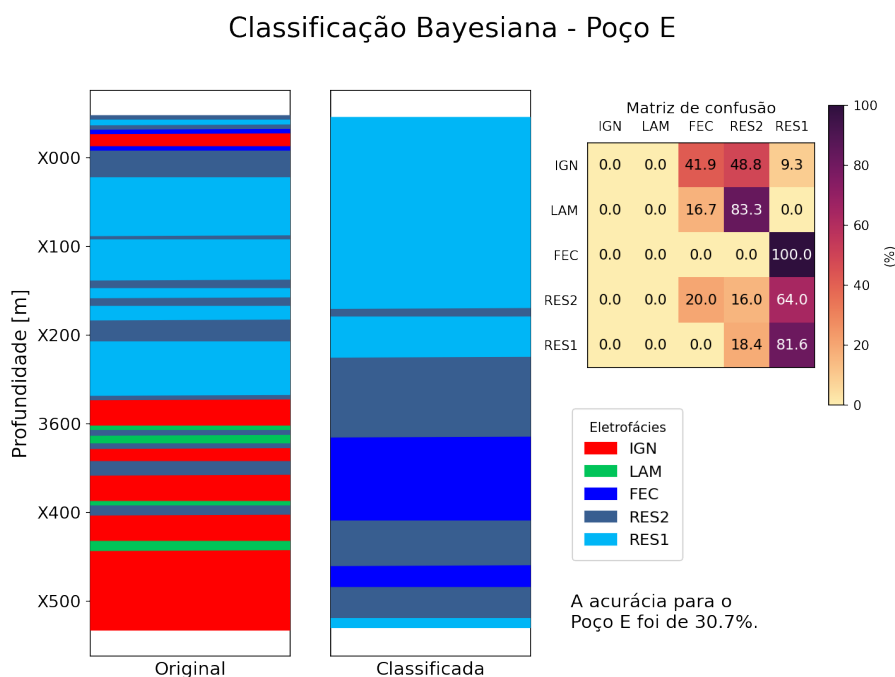
Figura 65 – Eletrofácies originais do Poço E e a extraída do volume classificado na posição do poço. Além disso, é mostrada a matriz de confusão e a acurácia estimada neste intervalo.
