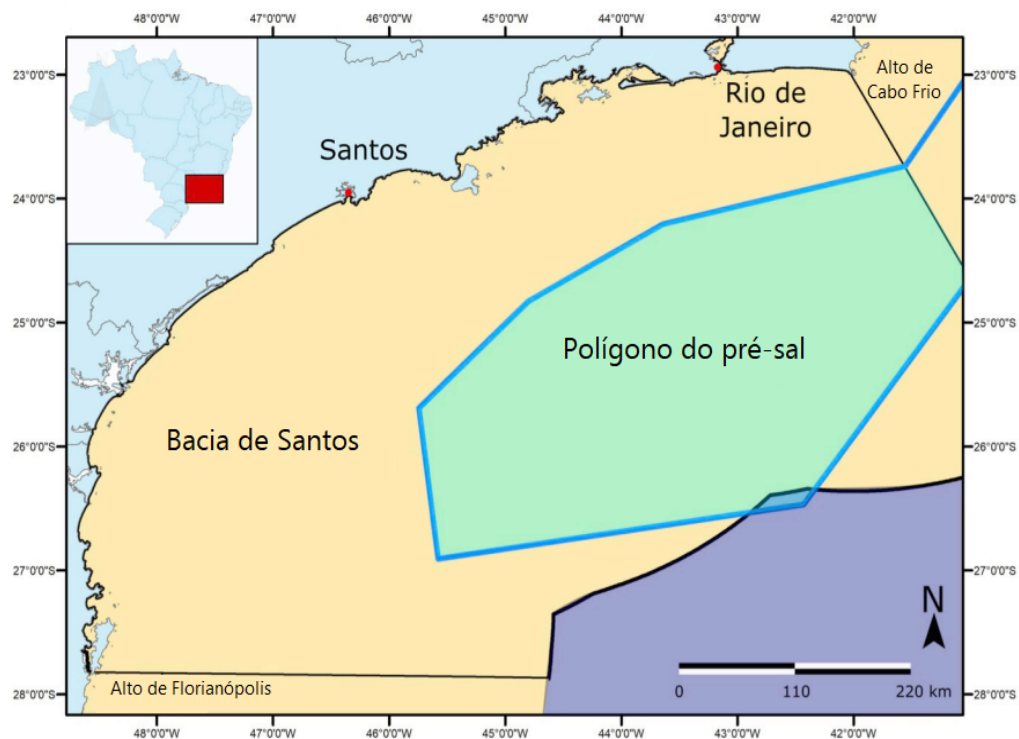
Figura 1 – Localização da Bacia de Santos, limitada pelo Alto de Florianópolis e o Alto de Cabo Frio, com o polígono do pré-sal em destaque. Modificado de Chinelatto et al. (2020) .
