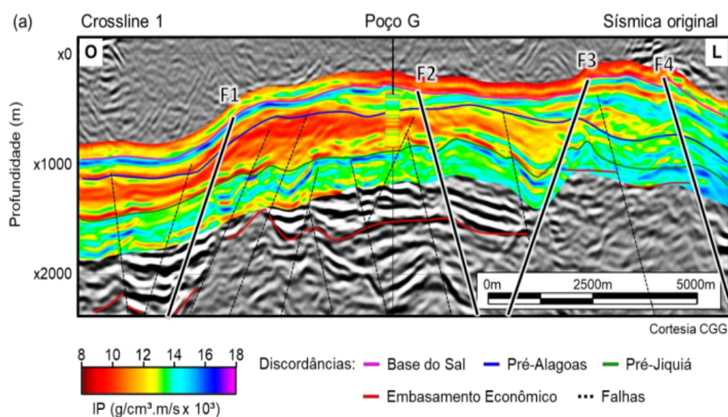
Figura 16 – Seção sísmica que corta o Poço G com a impedância acústica resultante da inversão determinística sobreposta ao dado sísmico. Fonte: Dias (2020).
