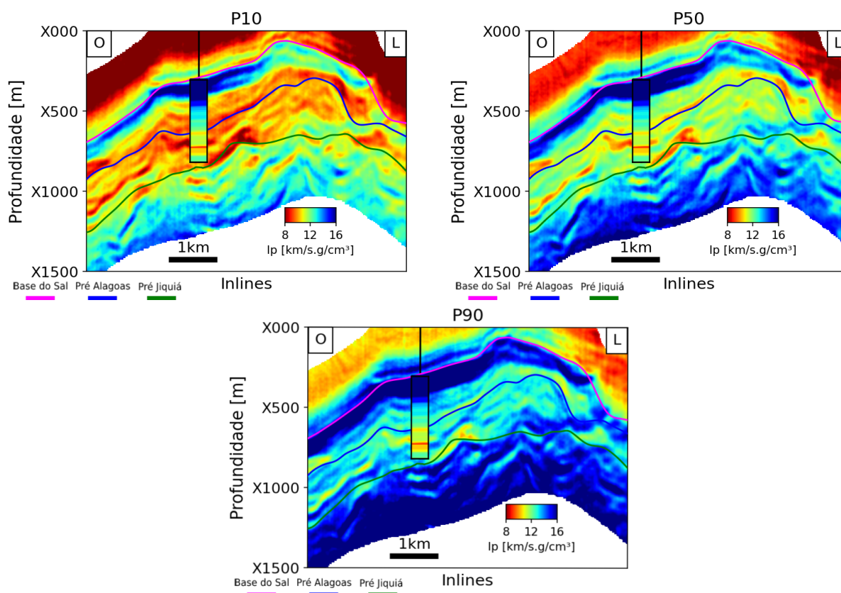
Figura 49 – Os três cenários gerados para a inversão estocástica na Seção sísmica 1. O P10 é mostrado acima na esquerda, o P50 acima na direita e o P90 abaixo.
