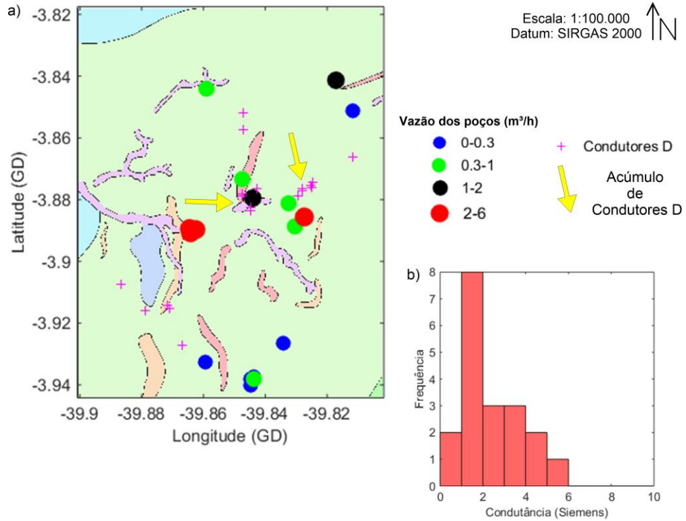
Figura 3: (a) Distribuição das fraturas (cruz em rosa) e poços cadastrados no SIAGAS. As setas amarelas indicam acúmulo de condutores, indicando possível relação com os poços próximos; (b) Histograma de Condutância (Siemens) para a anomalia do tipo D.
