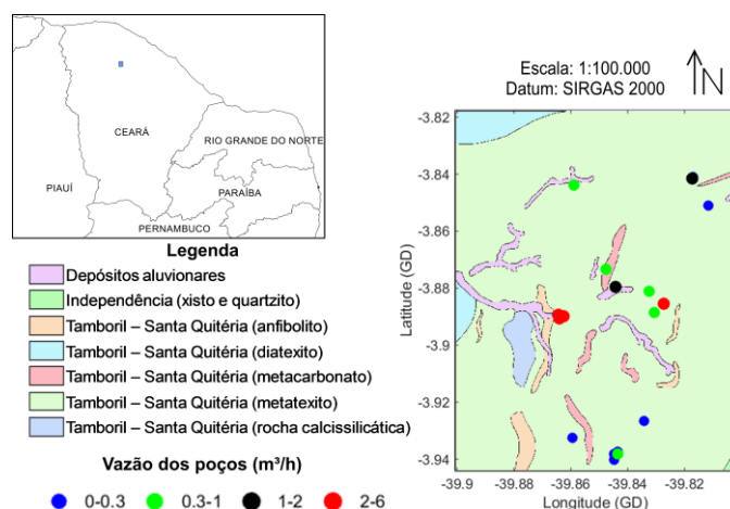
Figura 2: Localização e Geologia do Bloco Juá (CE) e dados de vazão de poços conforme cadastro do SIAGAS. Adaptado de CPRM – GEOBANK, Folha AS.24-Y-D-V-Iruçuaba.
