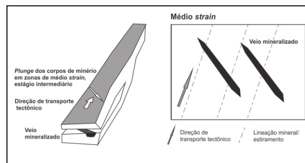
Figura 8 – Relações geométricas entre elementos estruturais e corpos de minério (eixos de dobras e boudins ). Com o aumento progressivo da deformação estes corpos tendem a rotacionar para o paralelismo com a direção de transporte tectônico (Adaptado e modificado de Robert & Poulsen, 2001).
