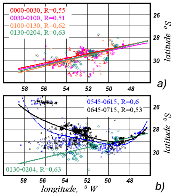
Figura 3 - Ajuste da posição da linha frontal pelo método dos quadrados mínimos usando acumulação dos raios durante 30 minutos: (a) 0000-0204 GMT de 27/07/99, estágio inicial; (b) estágio de maturidade do sistema 0545-0715 GMT com movimento do sistema ao norte. R são os coeficientes de correlação.
