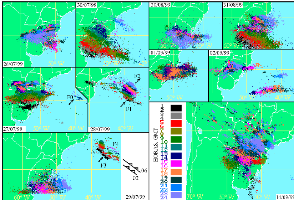
Figura 2 - Campos Acumulados das Descargas (CAD) durante ciclogênese local, dia 26/07/99, e desenvolvimento posterior da frente que move para interior do continente, no dia 27/07/99, precedendo a passagem da frente fria rápida nos dias 28/07/99 à 30/07/99. Linha da frente oceânica é marcada nas posições de F0 a F4 e é facilmente determinada durante os dias 27-29/07/99 (e.g. entre 0200 e 0600 GMT, 29/07/99). CAD da frente estacionária no dia 30/08/99; CAD durante ciclogênese frontal (31/08/99) e local (01/09/99-02/09/99, 14/09/99). O tempo é codificado em cores.
