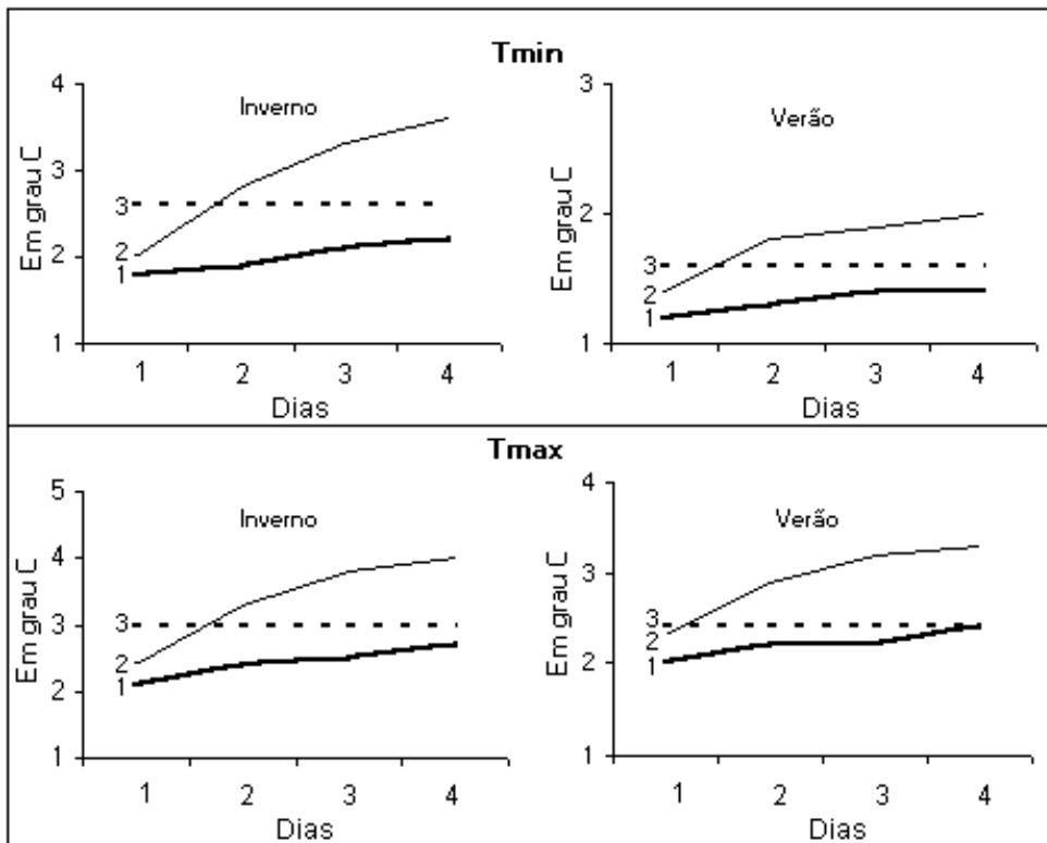
Figura 5 - Erro médio absoluto de previsões até 4 dias: 1 – MOS, 2 – persistência, 3 – climatologia.
