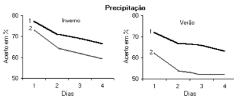
Figura 4 - Acerto das previsões de ocorrência de chuva: 1 – MOS, 2 – persistência.
