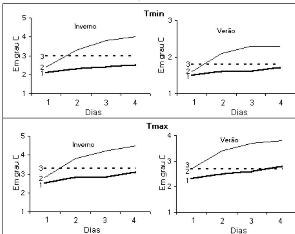
Figura 6 - Erro médio quadrático das previsões até 4 dias: 1 – MOS, 2 – persistência, 3 – climatologia.
