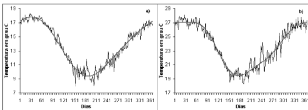
Figura 3 - Normas climáticas diárias da T_{\min} (a) e T_{\max} (b) e componentes cíclicas obtidas (negrito) na estação Ponta Grossa.
