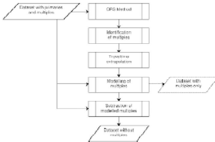
Figure 4 – The method considered for the multiple attenuation by modelling, using CRS parameters, involves: (a) Identification of multiples, (b) modelling of multiple in any domain and adjust the amplitudes, and (c) subtraction of multiples. Figura 4 – O método considerado para a atenuação de múltiplas por modelando, usando os parâmetros do CRS, envolve: (a) Identificação das múltiplas, (b) modelamento das múltiplas em algum domínio e ajuste das amplitudes, e (c) subtração das múltiplas.
