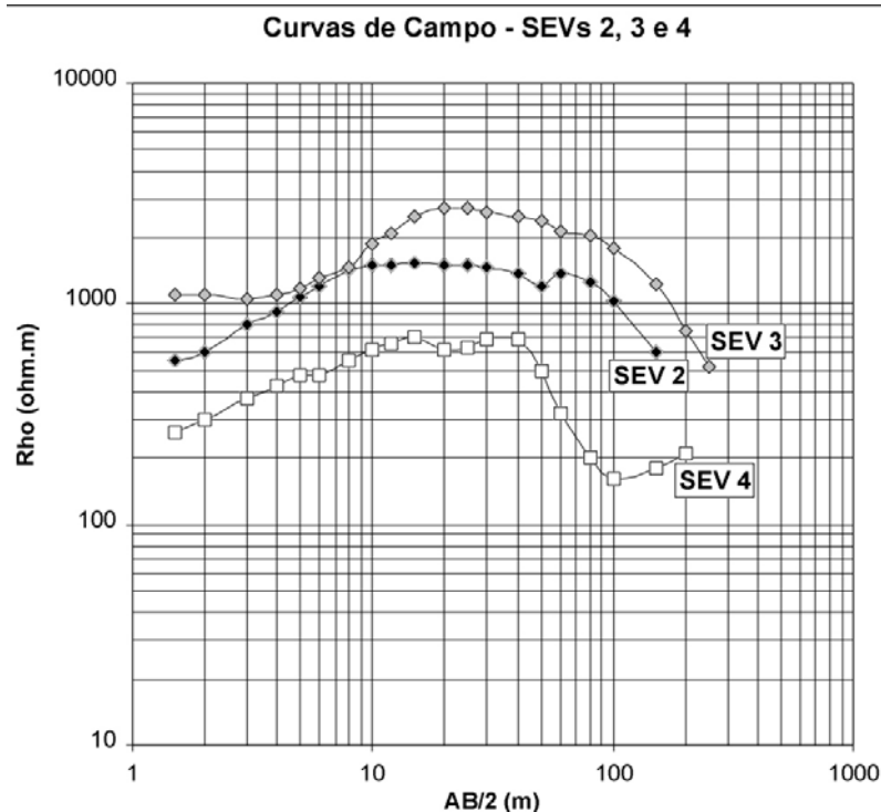
Figura 6 – Curvas de campo das SEVs 2, 3 e 4.
