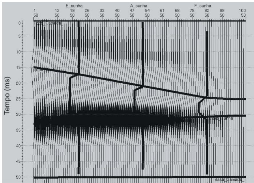
Figura 6 – Modelo integrado apresentando os horizontes interpretados no dado sísmico que constituem o modelo estrutural do reservatório de referência.
