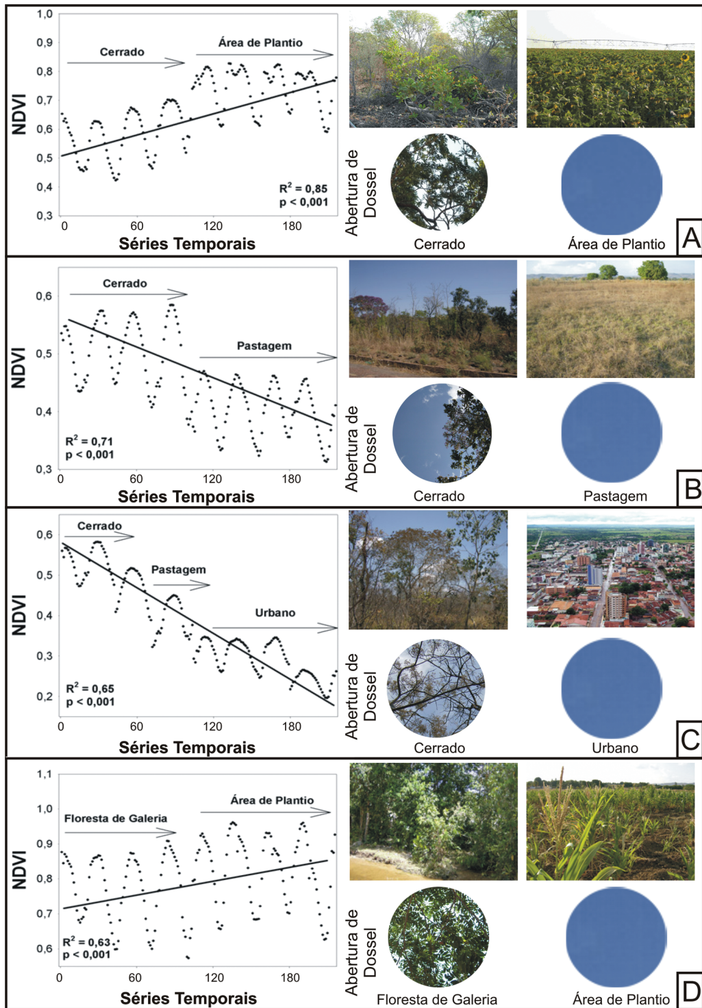
Figura 4 – Relação dos valores índice de vegetação NDVI de janeiro de 2000 a dezembro de 2008 (a cada 16 dias), dos pixels que obtiveram mudança de Cerrado a Área de Plantio (4A) 16°21'03,52''S e 46°56'11,80''O; de Cerrado a Pastagem (4B) 16°20'34,56''S e 46°57'48,73''O; de Cerrado a Área Urbana (Unai/MG) (4C) 16°20'59,25''S e 46°54'47,87''O; e de Floresta de Galeria a Área de Plantio (4D) 16°00'47,64''S e 47°06'52,98''O; na área da Bacia do Rio Paracatu. A reta representa o ajuste linear ( R^2 = coeficiente de determinação e p = nível de significância). Fotos e abertura de dossel representativos da área de mudança temporal.
